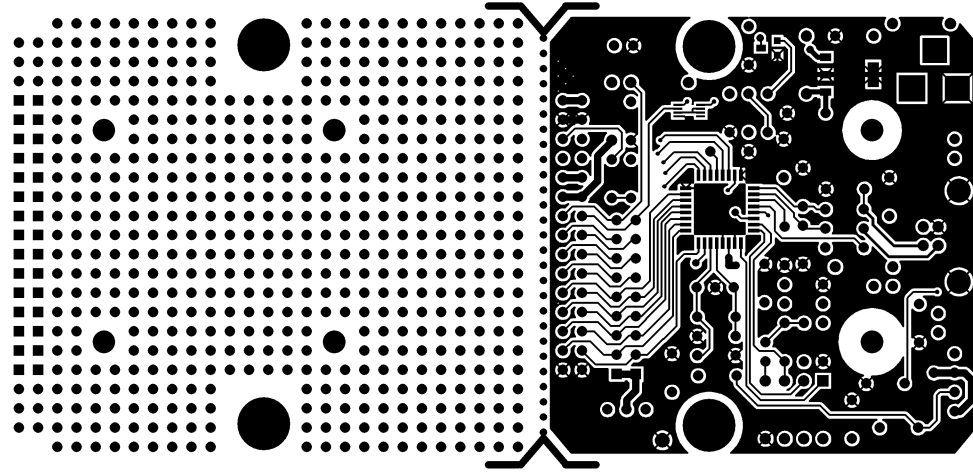
TOP LAYER
