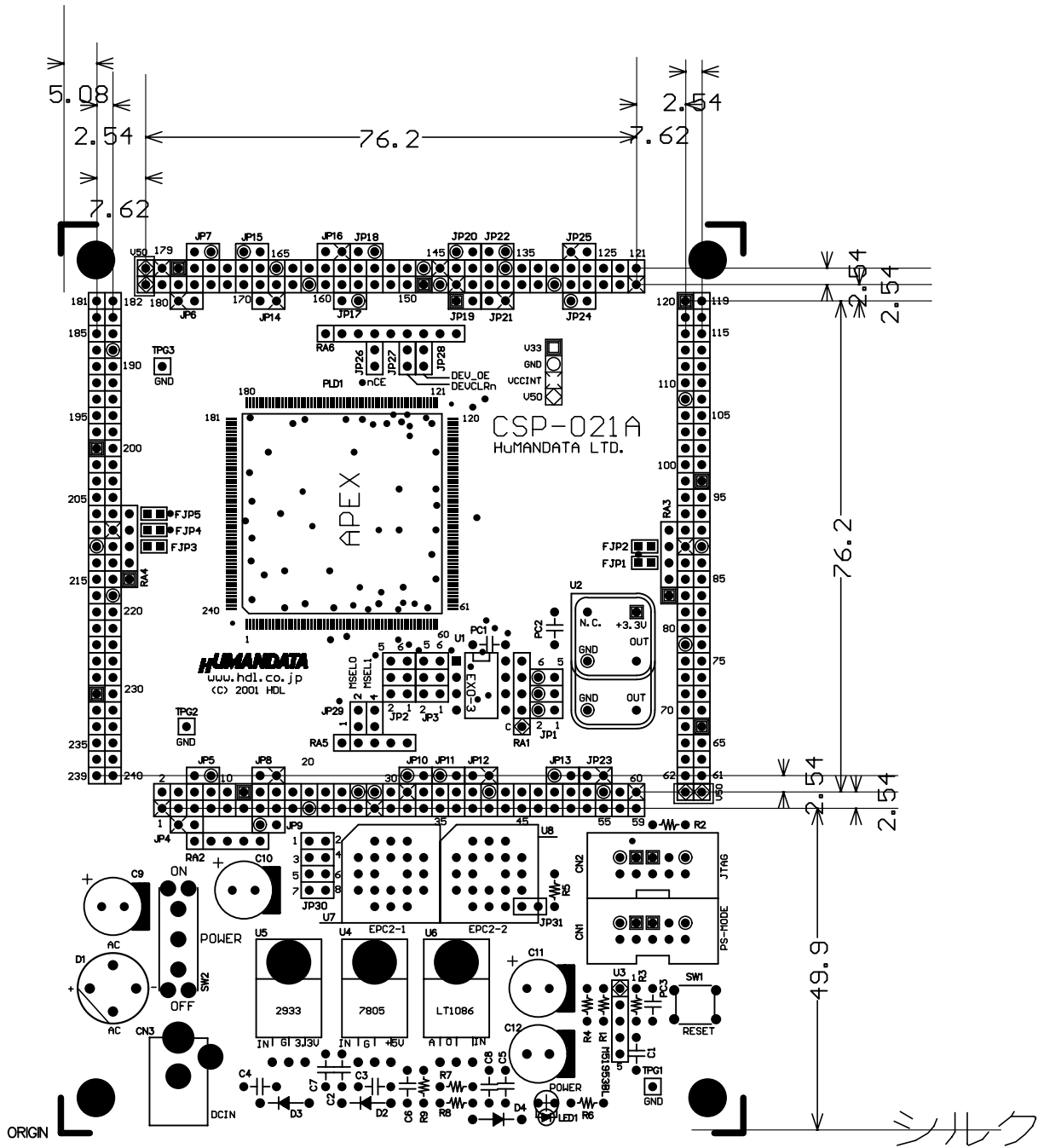
Top Overlay
