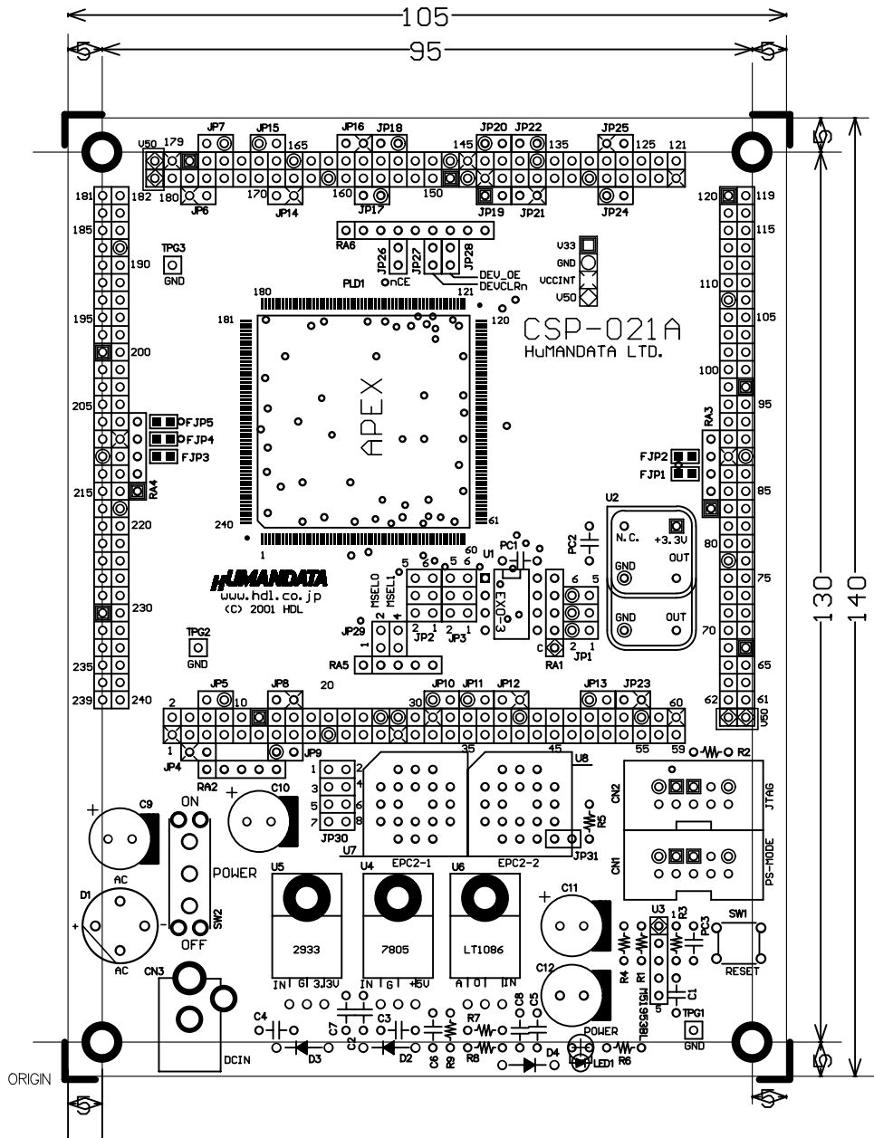
Top Overlay
