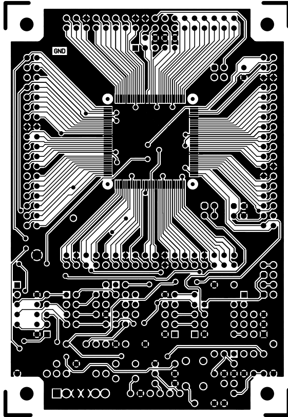
Top Layer
