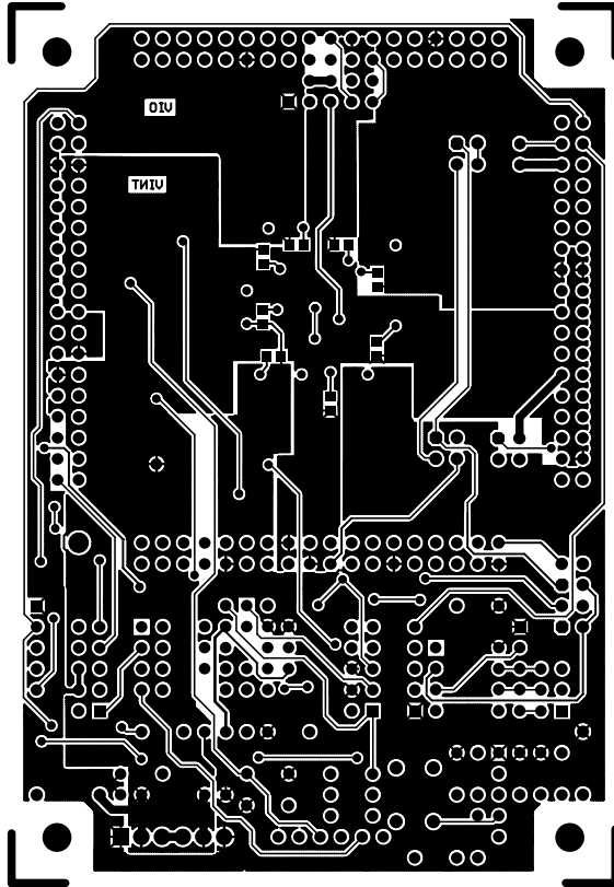
Bottom Layer
