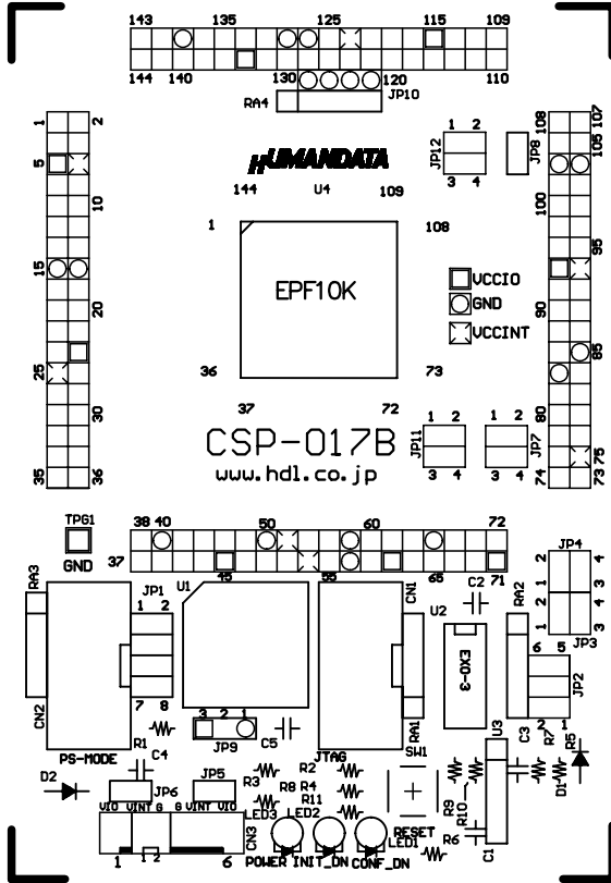
Top Overlay
