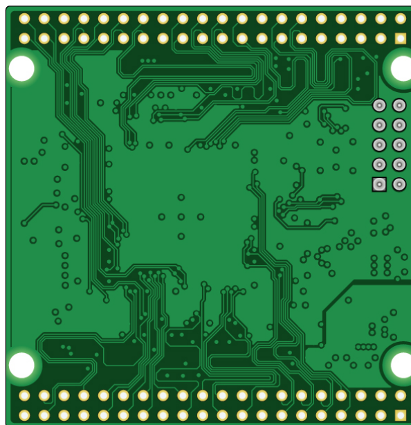
はんだ面
