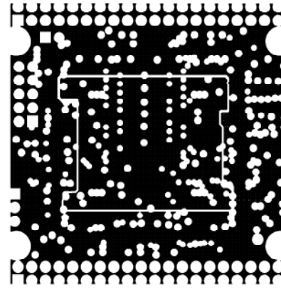
MID LAYER2
