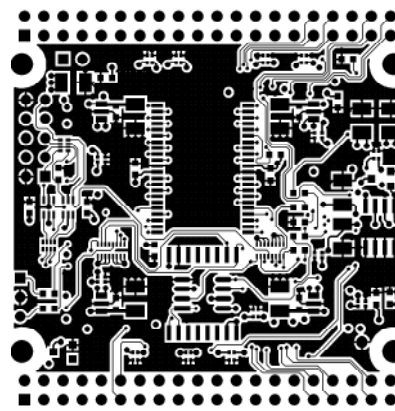
BOTTOM LAYER
