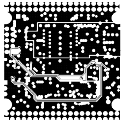
MID LAYER1
