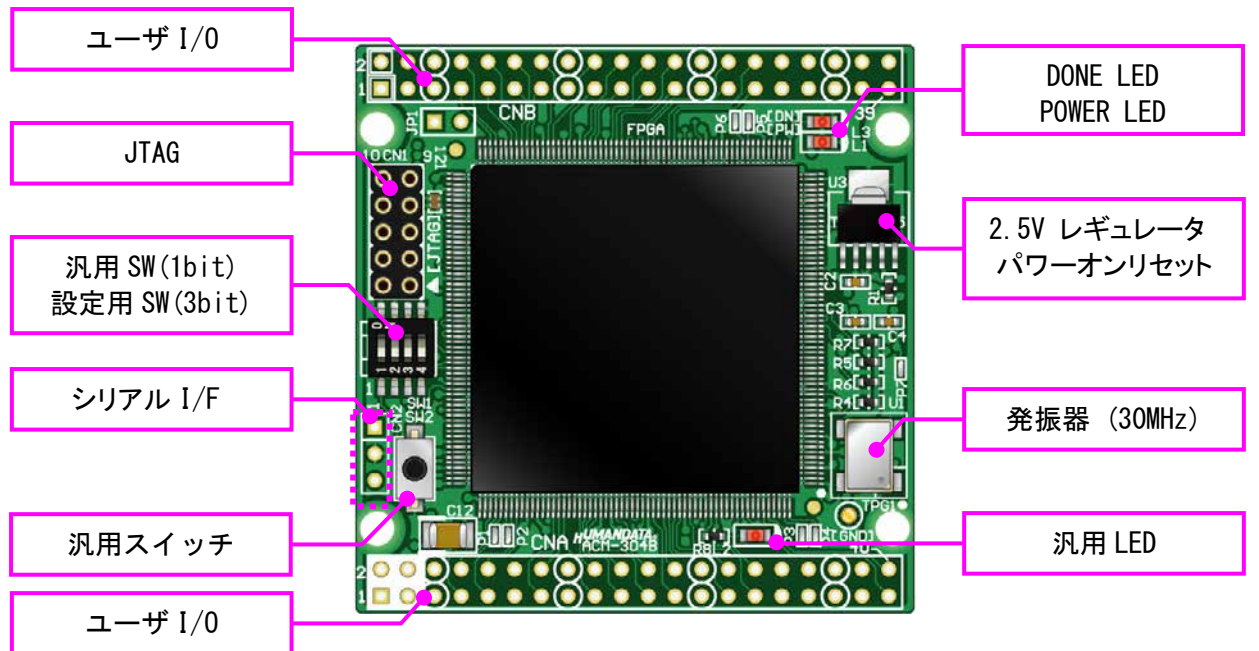
部品面
