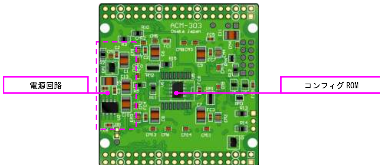
はんだ面
