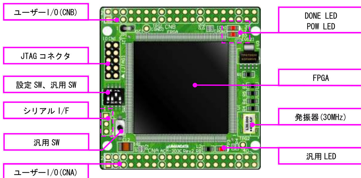
部品面
