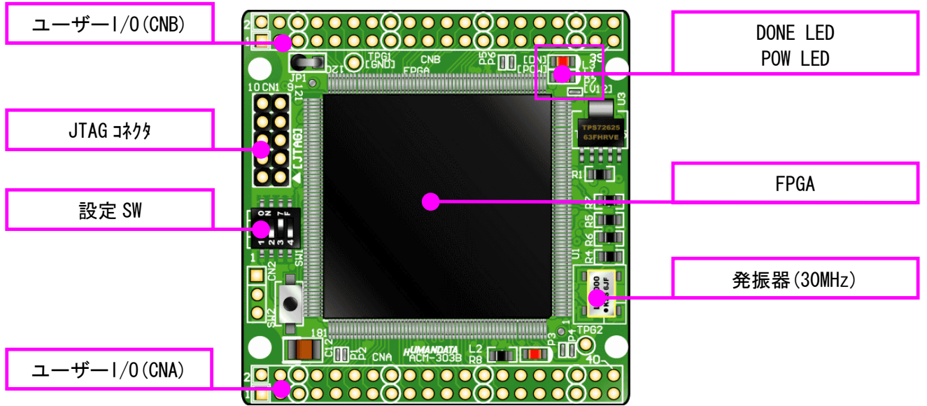
部品面
