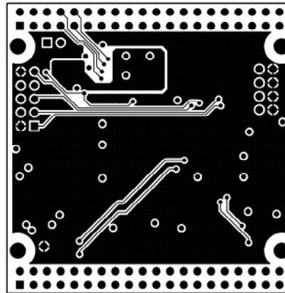
BOTTOM LAYER
