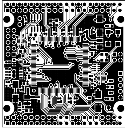
TOP LAYER
