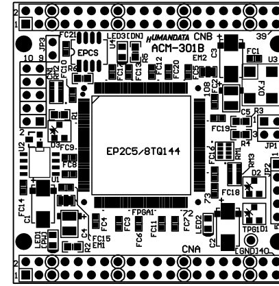
部品面
