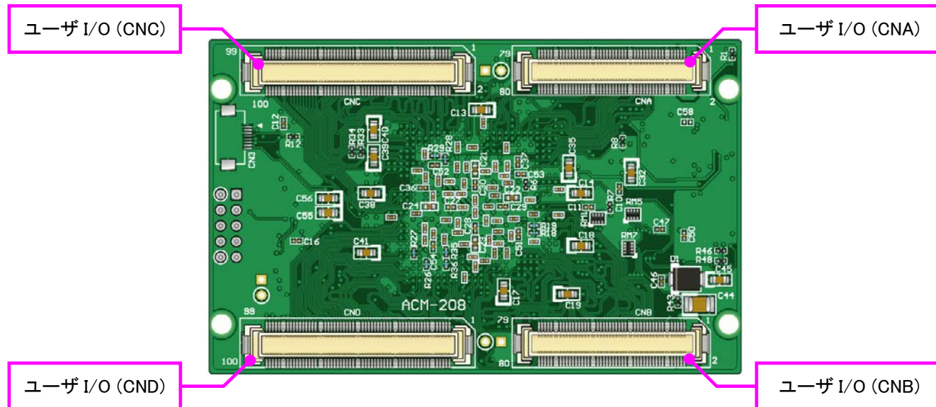
はんだ面
