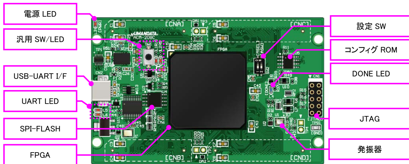
部品面
