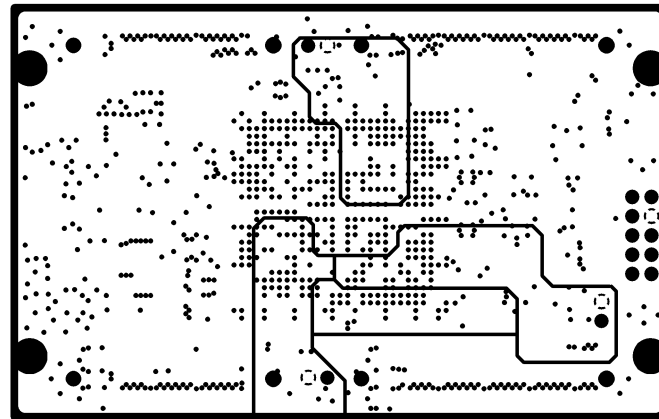
MID LAYER 1
