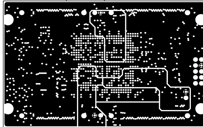
Internal Plane3 (Scale 1:1)
