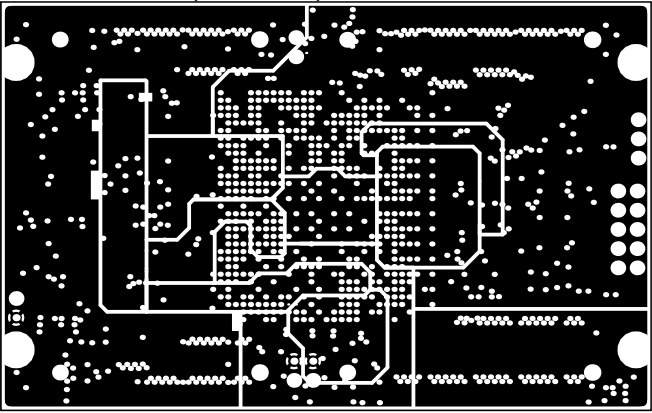
InternalPlane4 (Scale 1:1)
