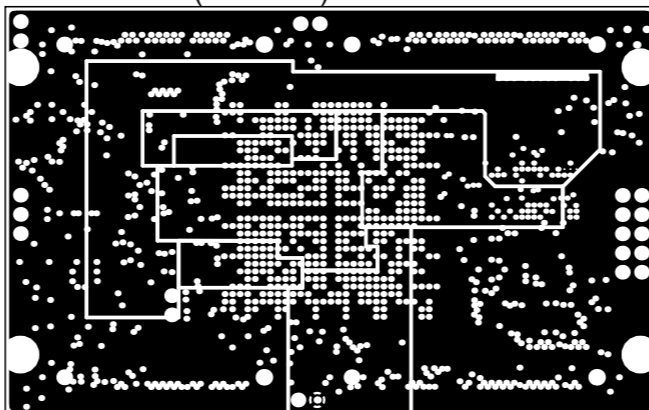
InternalPlane4 (Scale 1:1)
