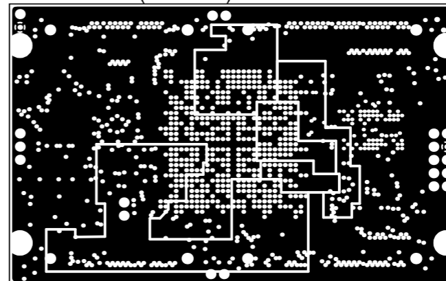
InternalPlane2 (Scale 1:1)
