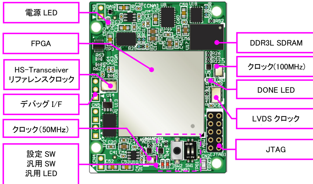
部品面
