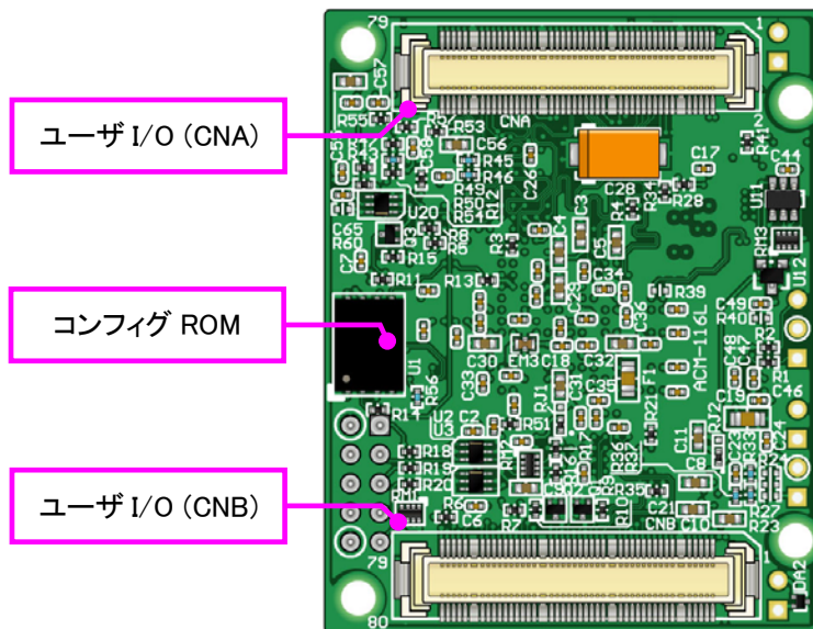
はんだ面
