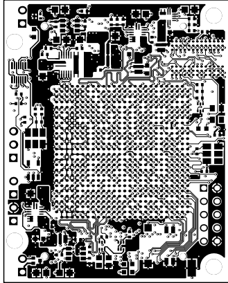
Top Layer (Scale 1:1)
