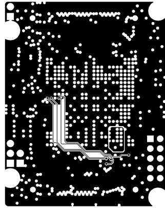
MID LAYER1
