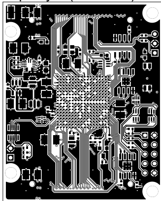
Top Layer (Scale 1:1)
