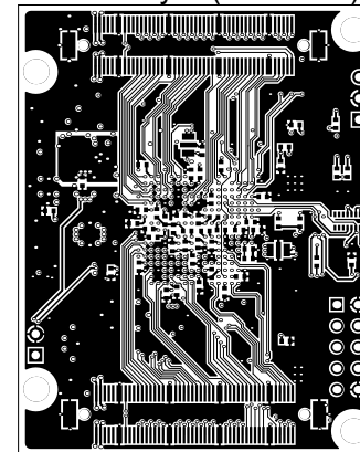
Bottom Layer (Scale 1:1)
