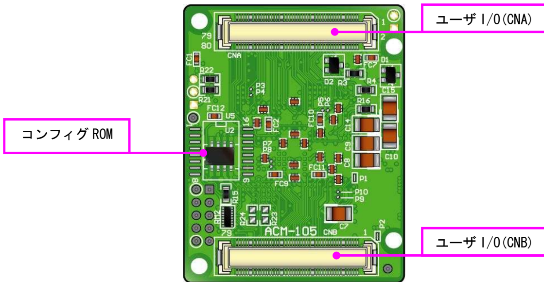
はんだ面
