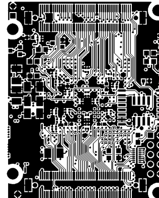
BOTTOM LAYER
