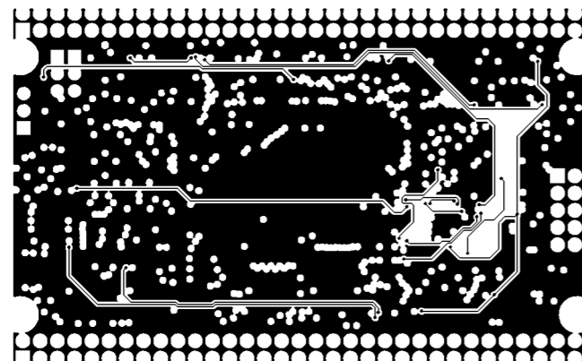
MID LAYER1
