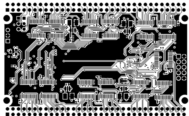
BOTTOM LAYER
