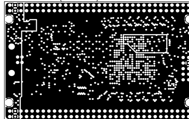
InternalPlane2 (Scale 1:1)
