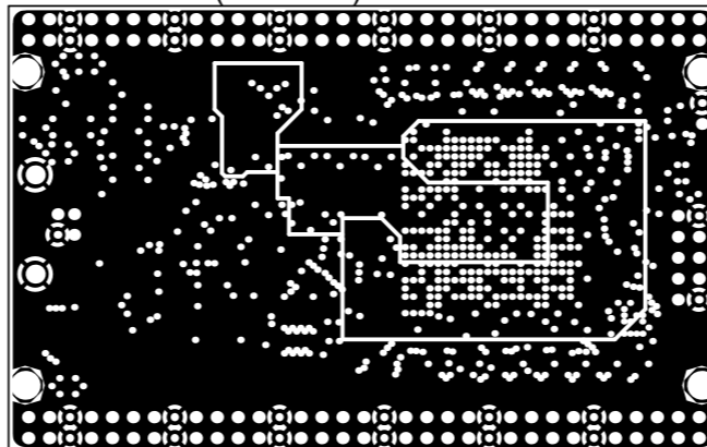
InternalPlane3 (Scale 1:1)
