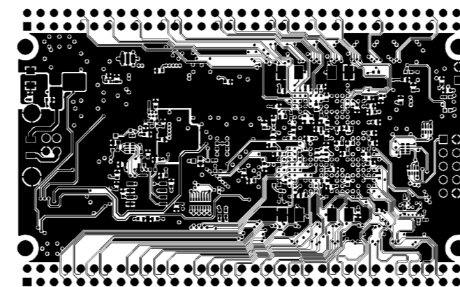
BOTTOM LAYER
