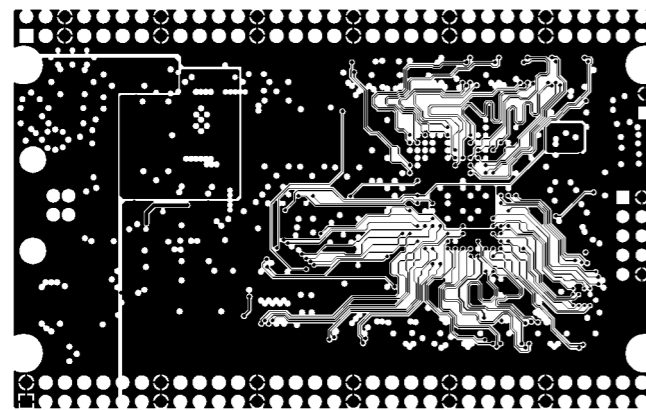
MID LAYER1
