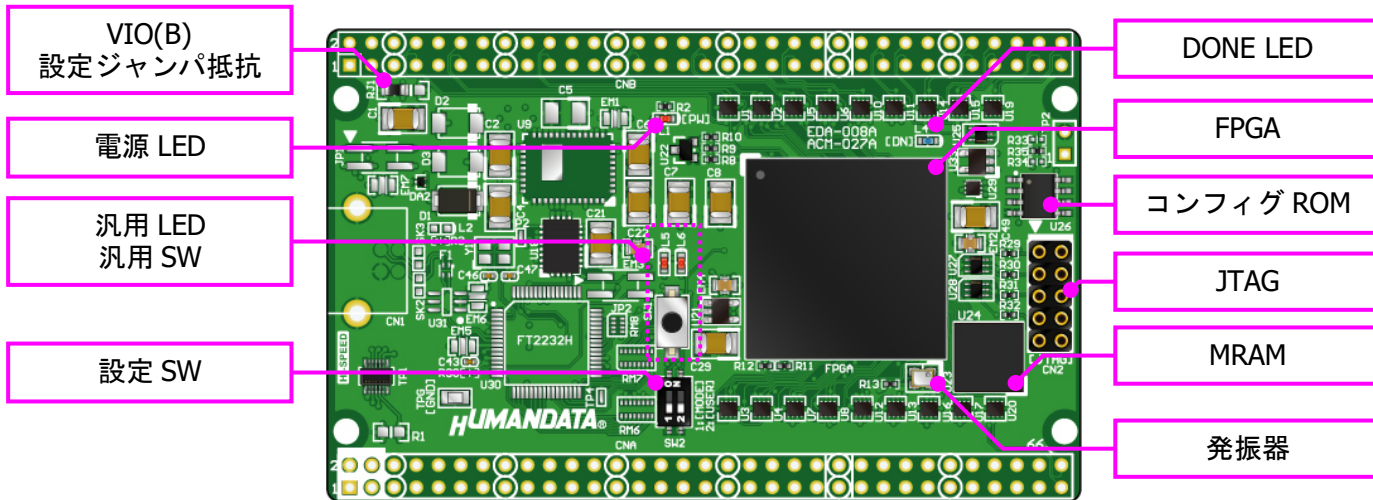
部品面
