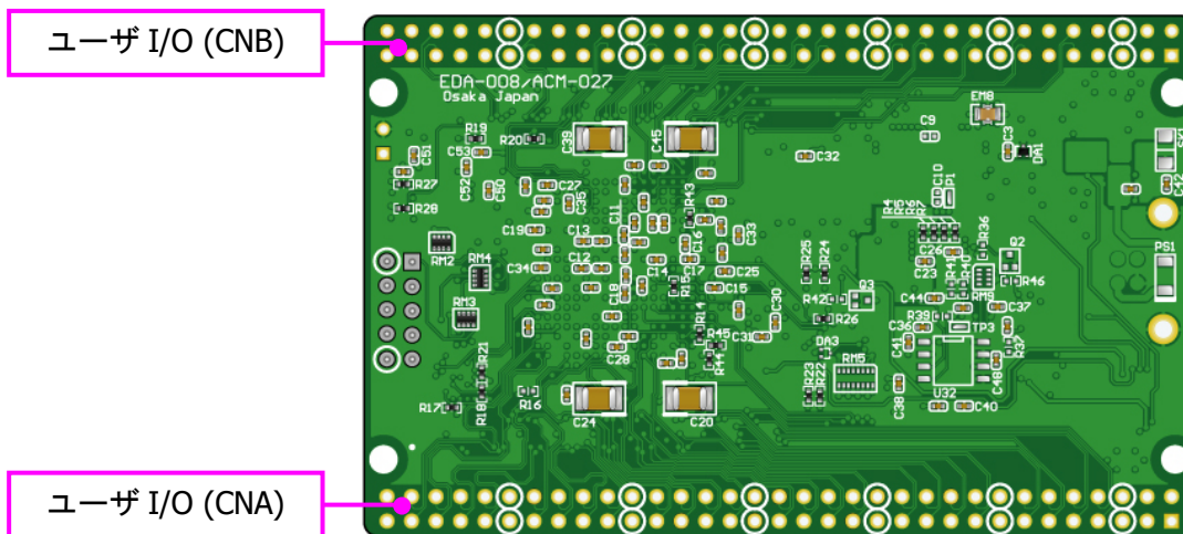
はんだ面
