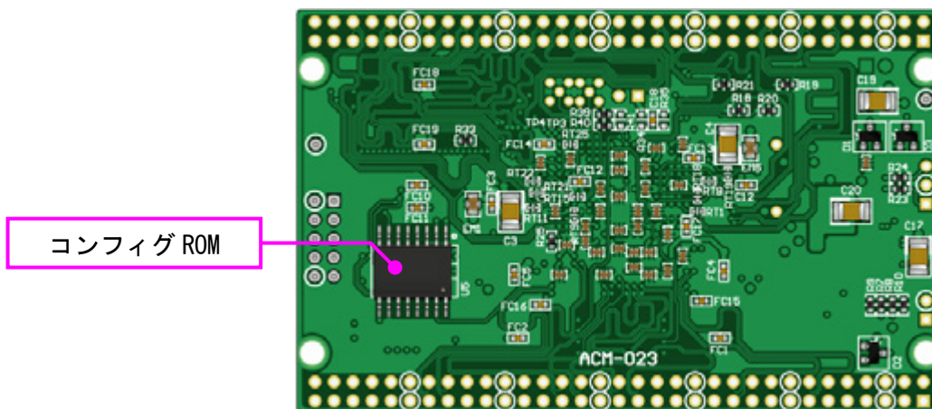
はんだ面
