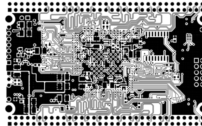
BOTTOM LAYER
