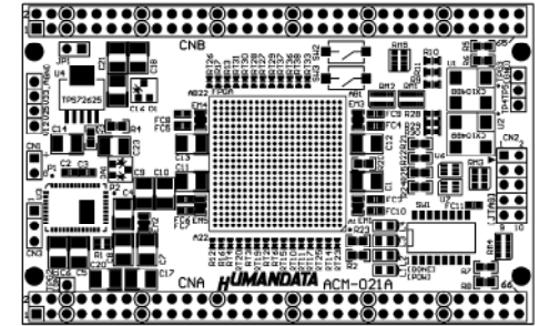
部品面
