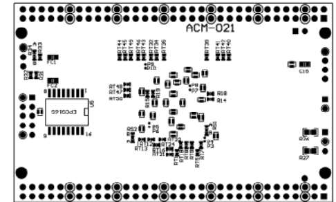
はんだ面
