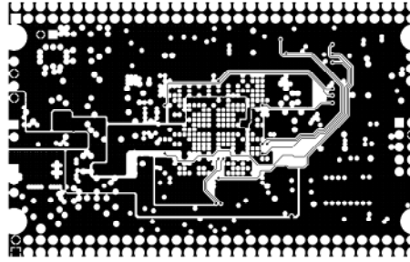
MID LAYER2
