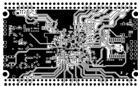
BOTTOM LAYER
