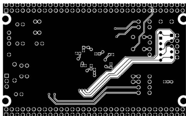
BOTTOM LAYER
