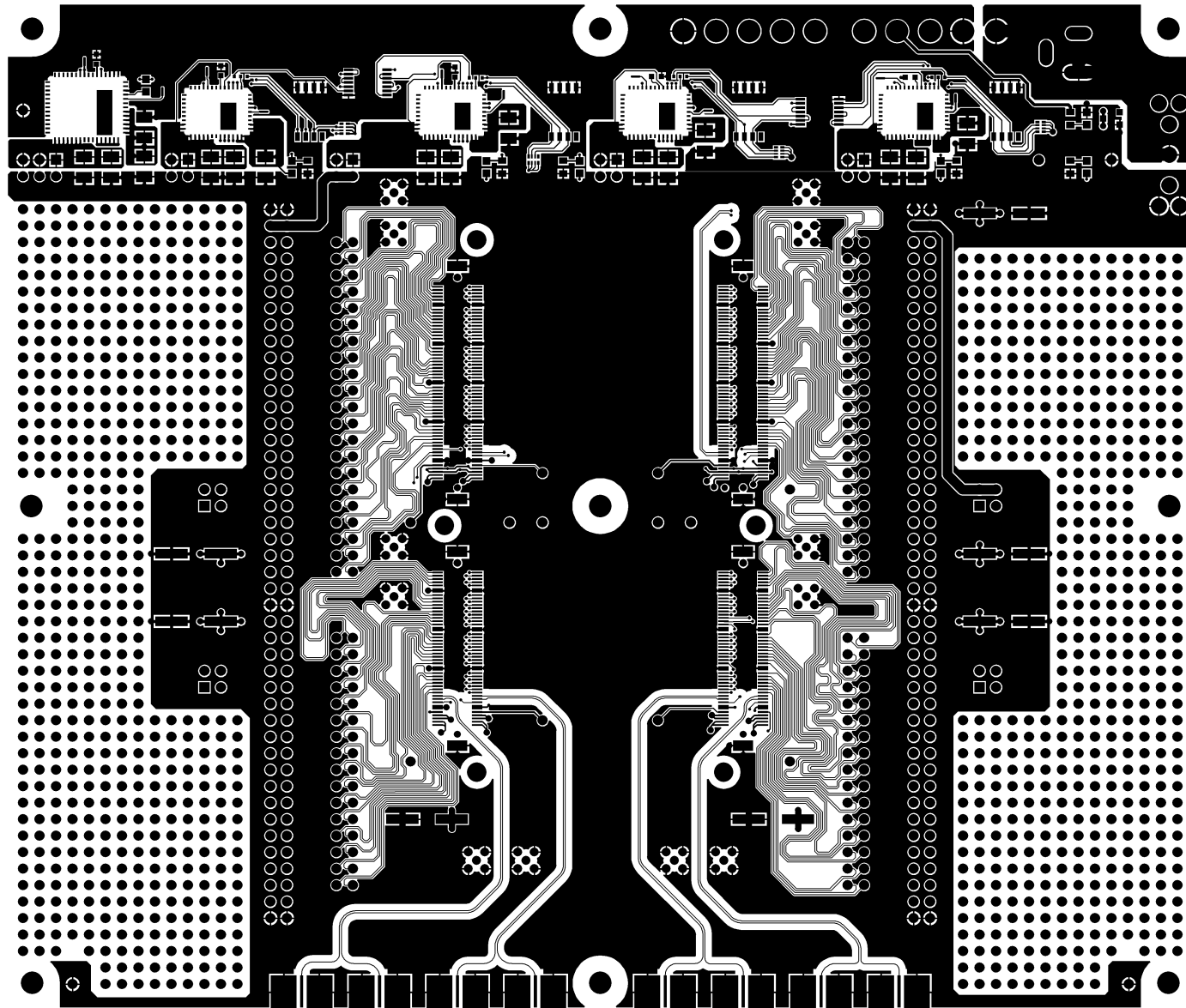
TOP LAYER
