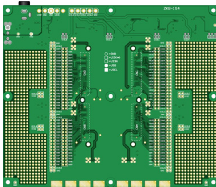
はんだ面 (部品実装はありません)
