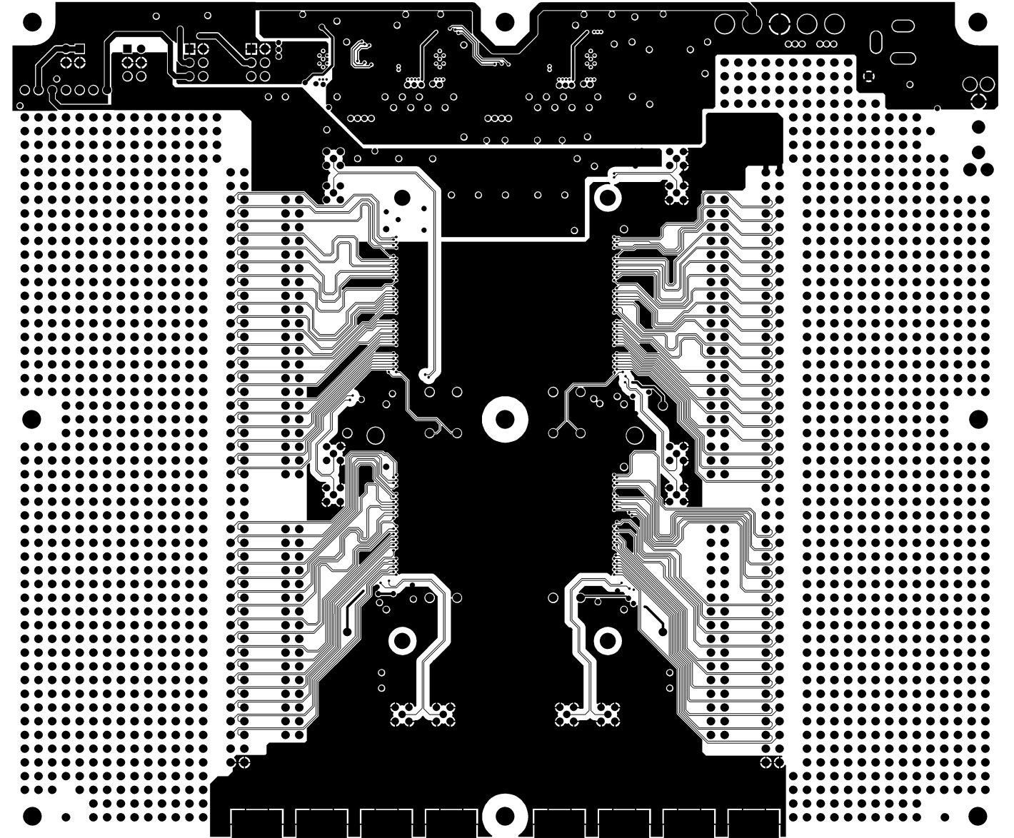
BOTTOM LAYER
