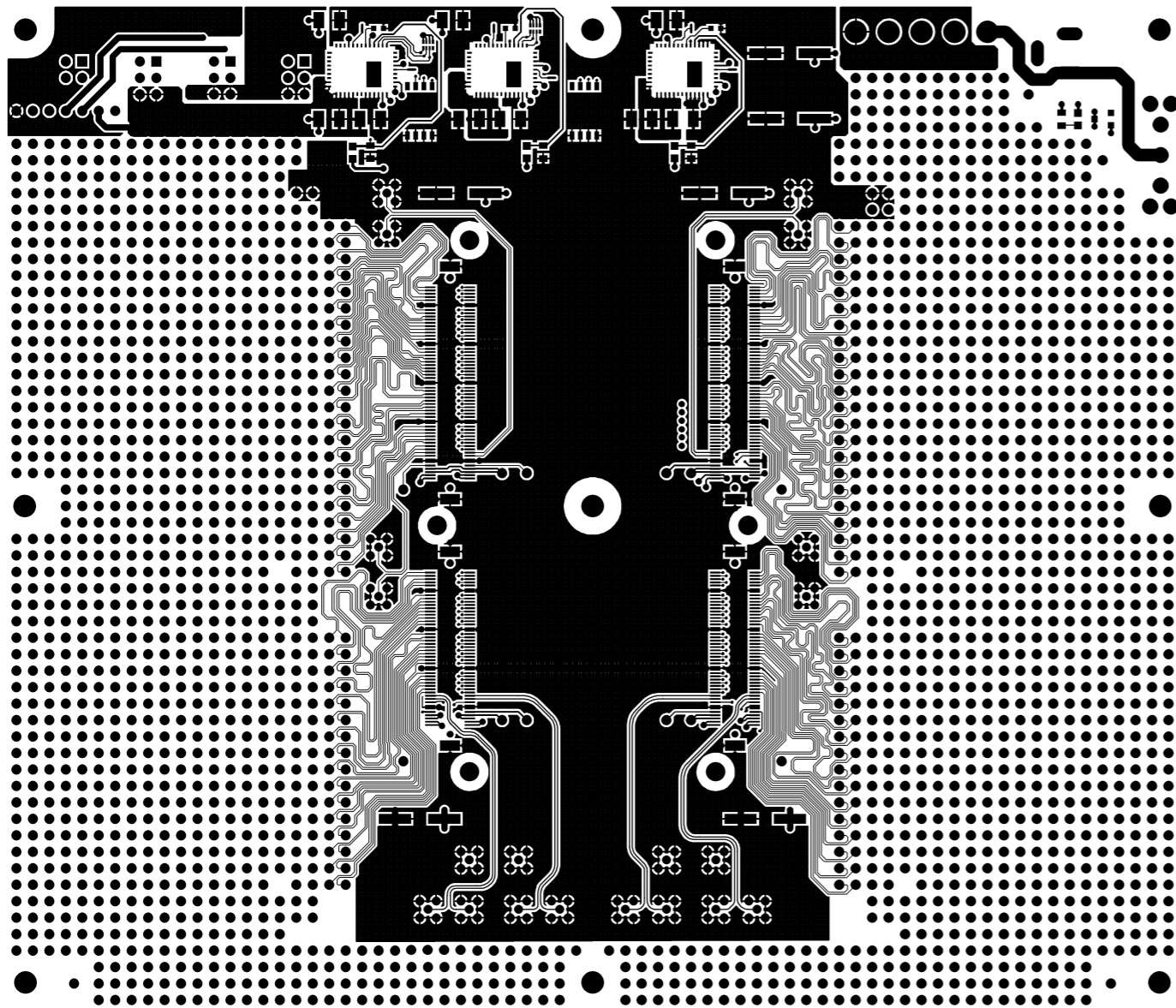
TOP LAYER
