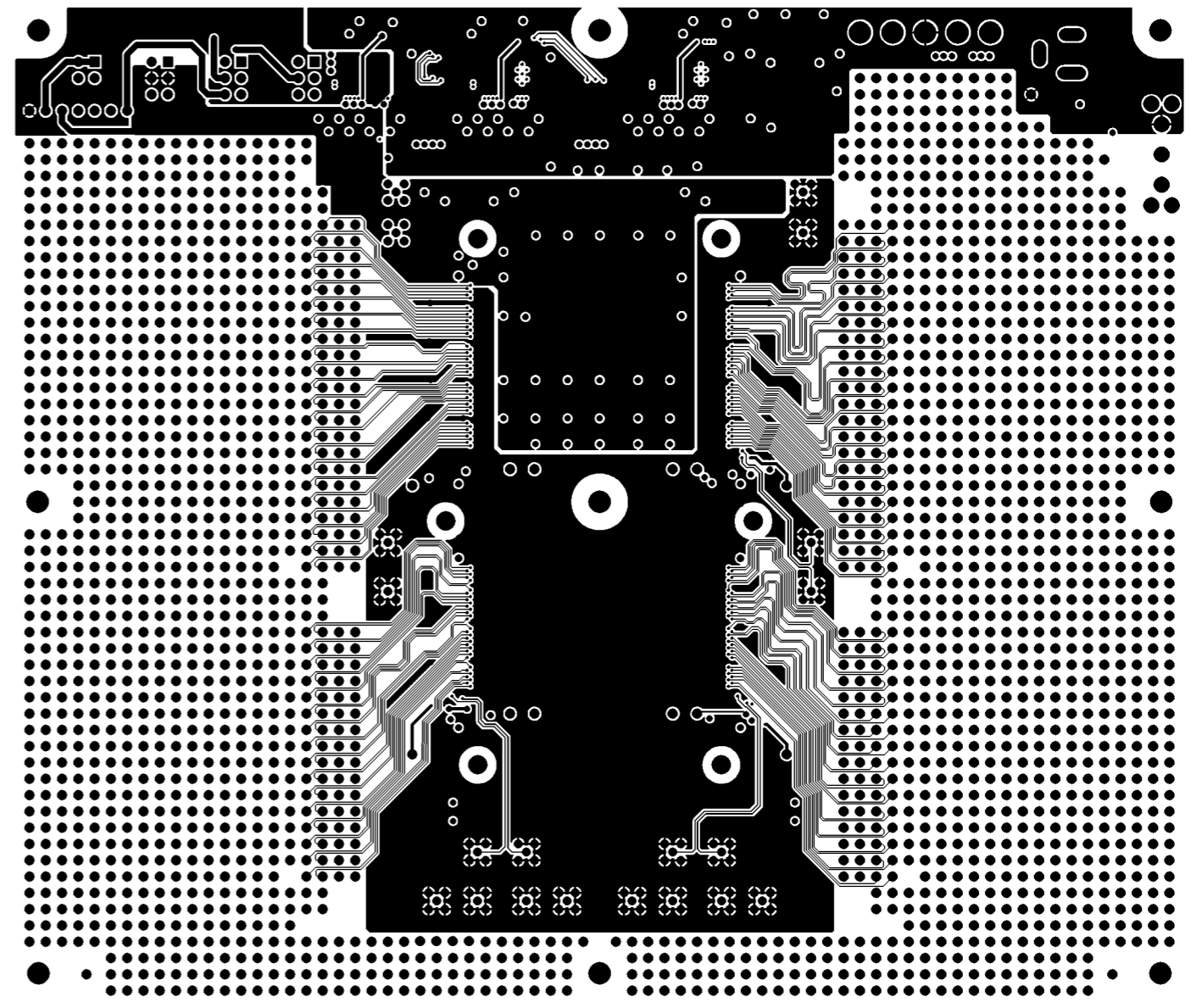
BOTTOM LAYER
