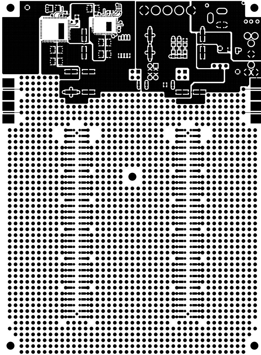
TOP LAYER
