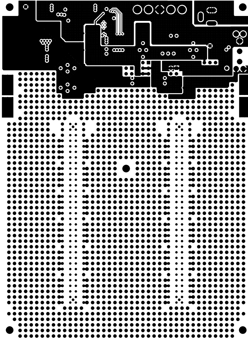
BOTTOM LAYER
