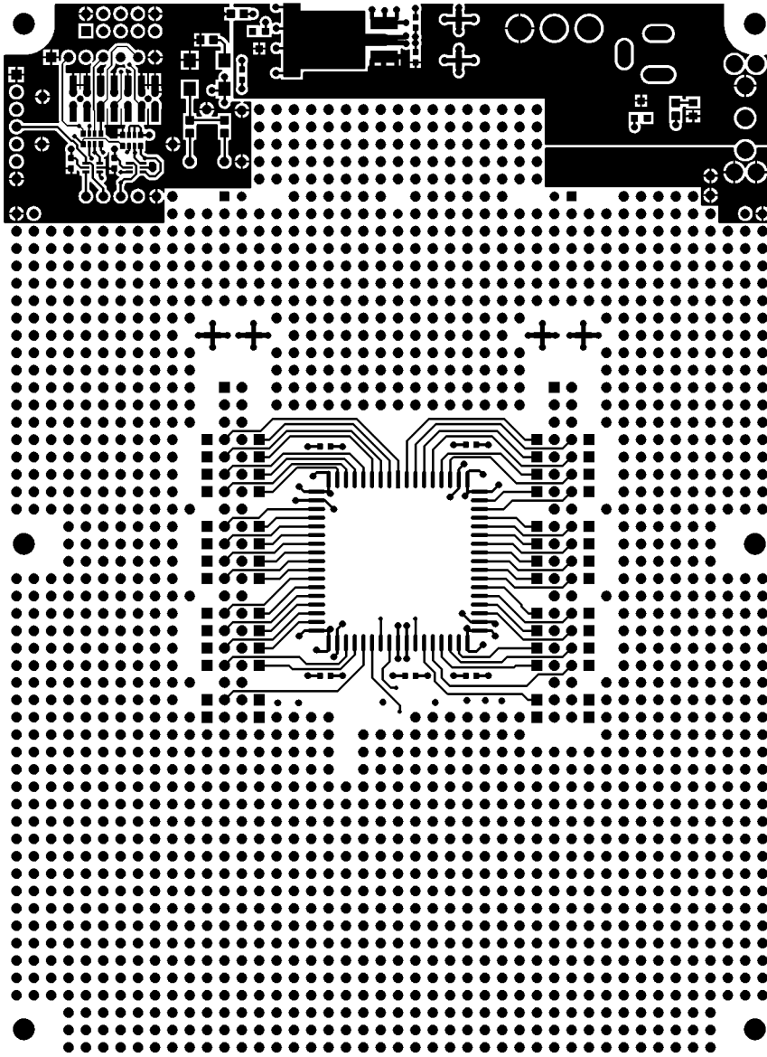
TOP LAYER
