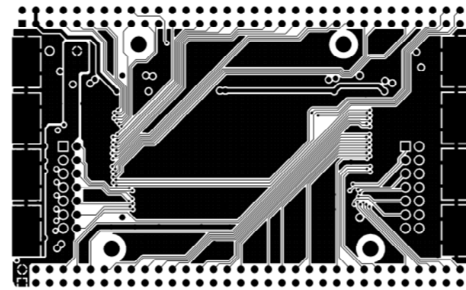
BOTTOM LAYER
