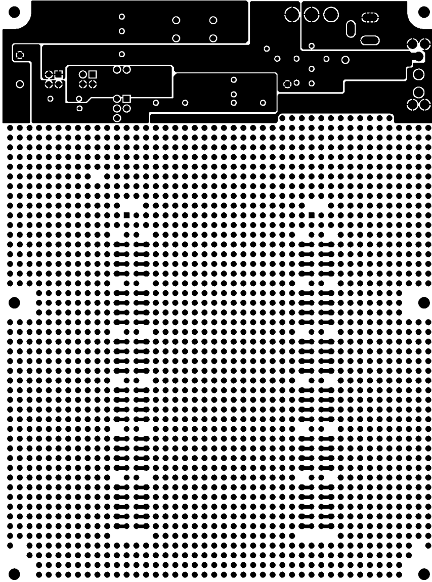
BOTTOM LAYER
