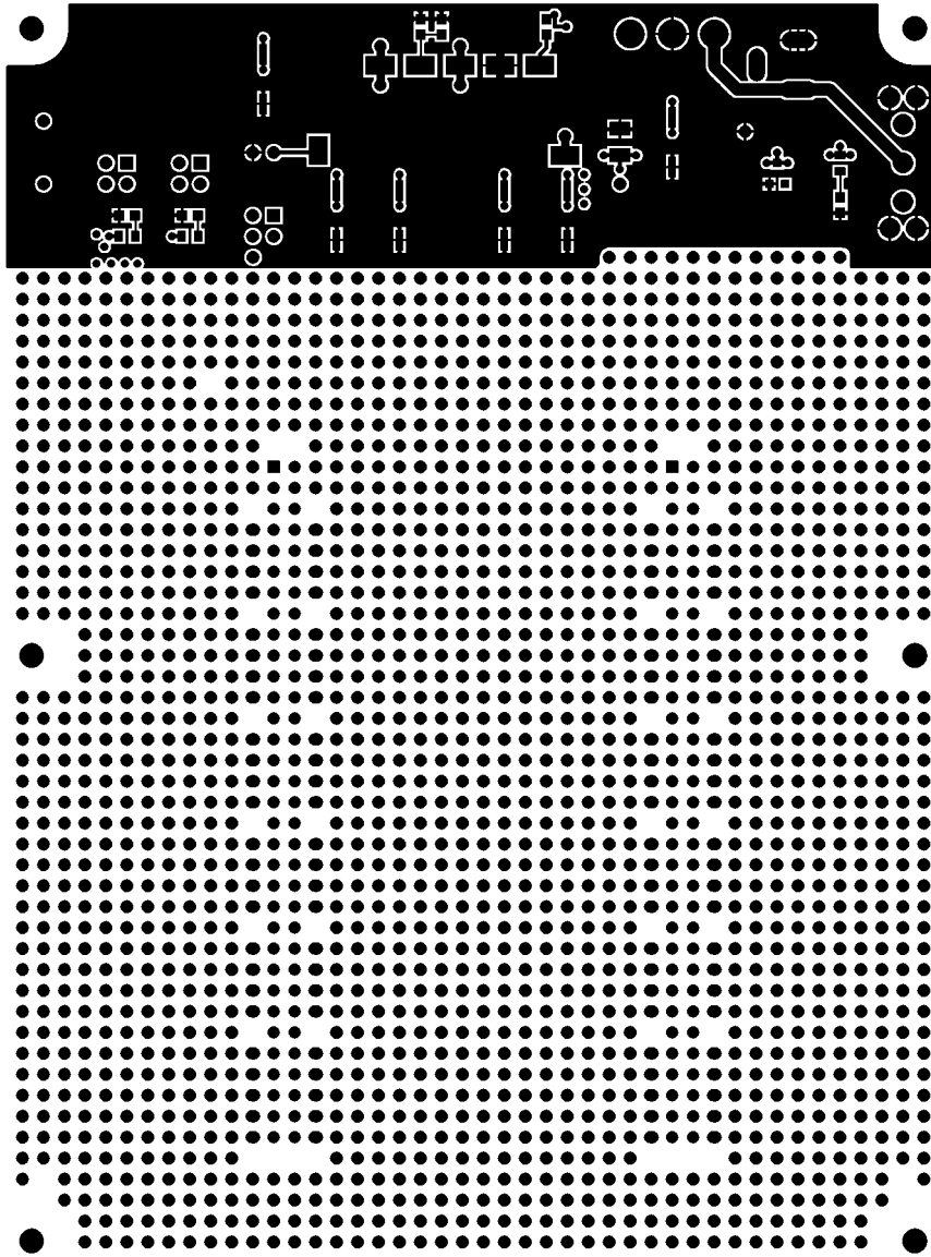
TOP LAYER
