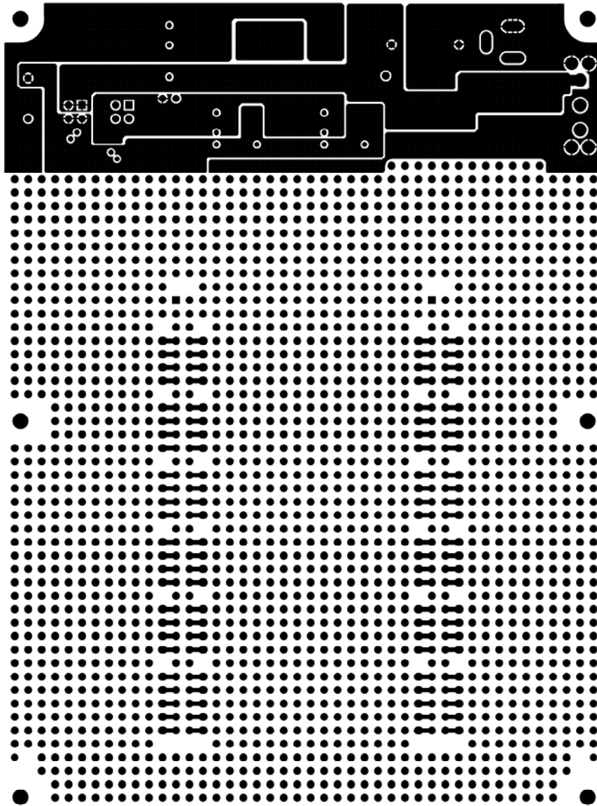
BOTTOM LAYER
