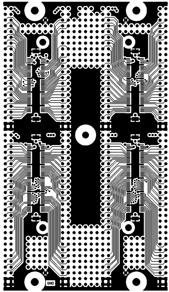
TOP LAYER
