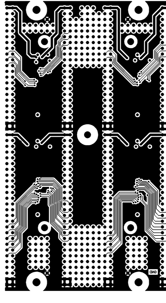
BOTTOM LAYER
