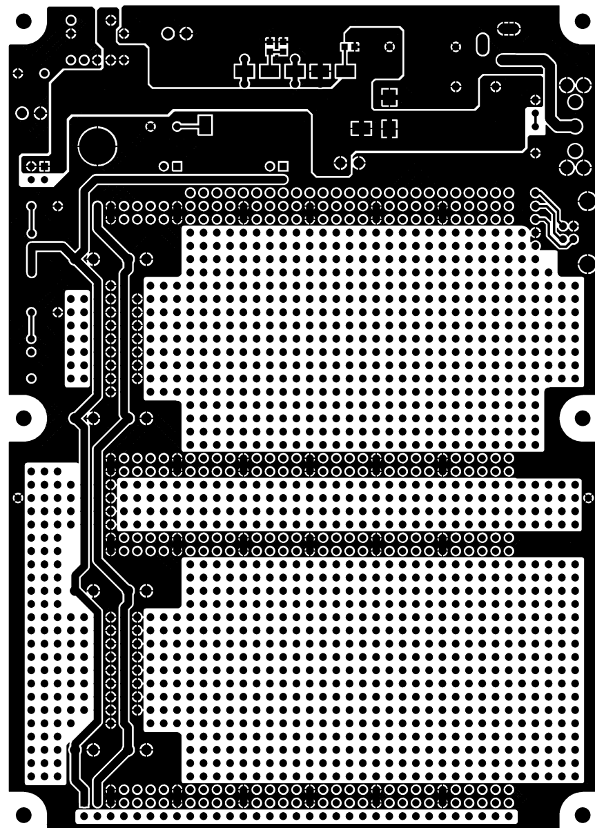
TOP LAYER
