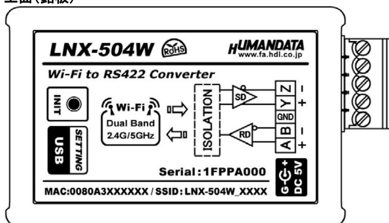
上面(銘板)
