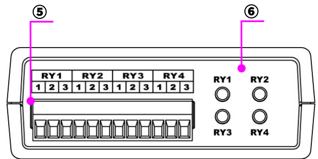
Photo リレー出力側パネル
