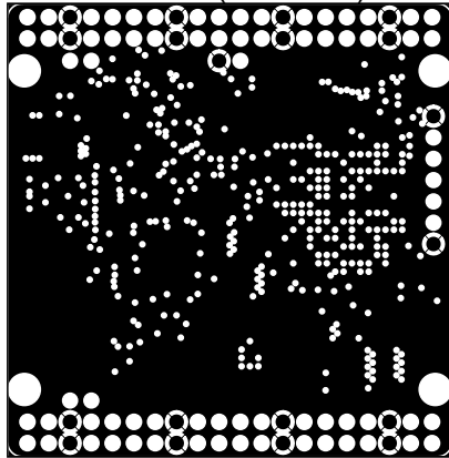
InternalPlane1 (Scale 1:1)
