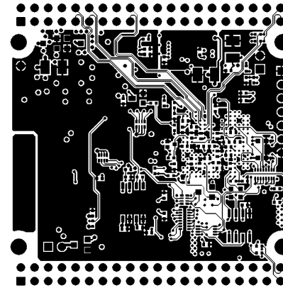
BOTTOM LAYER
