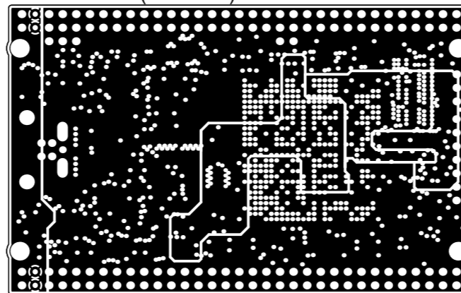
InternalPlane4 (Scale 1:1)
