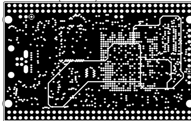
InternalPlane3 (Scale 1:1)
