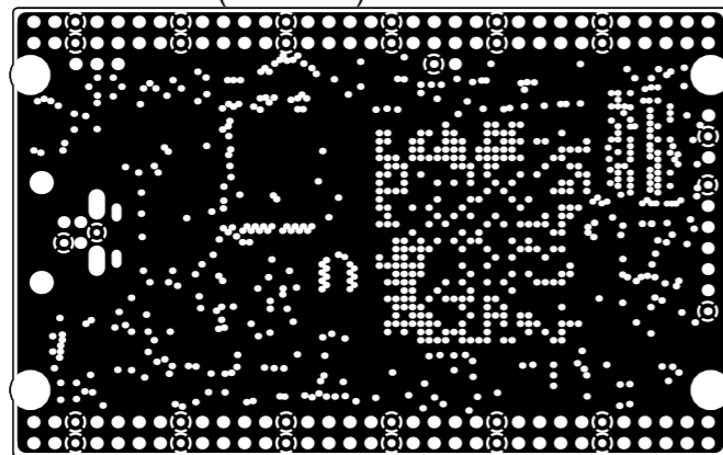
InternalPlane1 (Scale 1:1)
