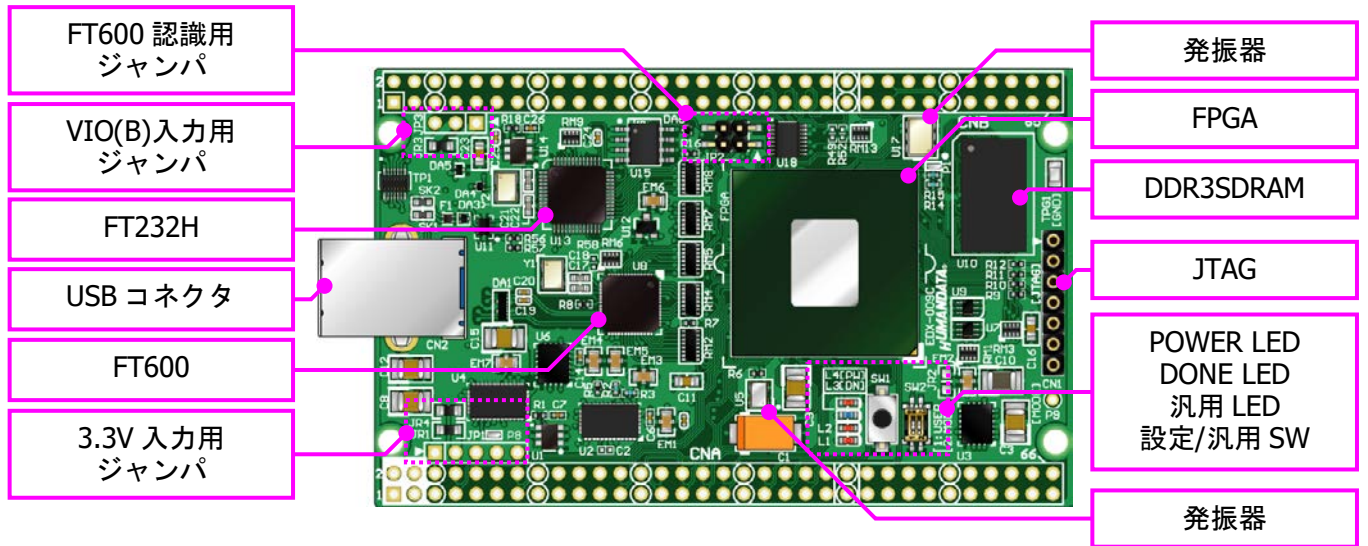
部品面
