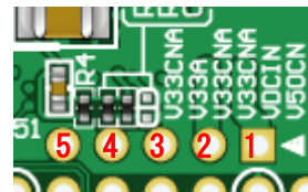
【はんだ面】
