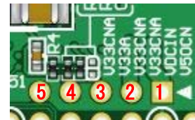
【はんだ面】
