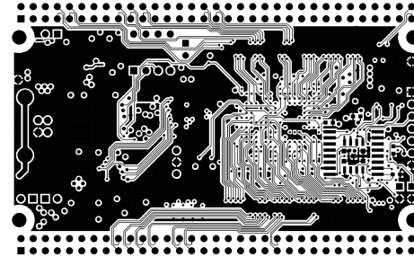
BOTTOM LAYER
