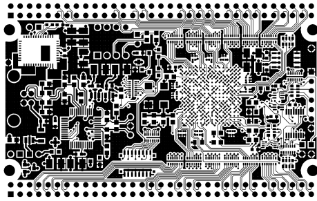
TOP LAYER
