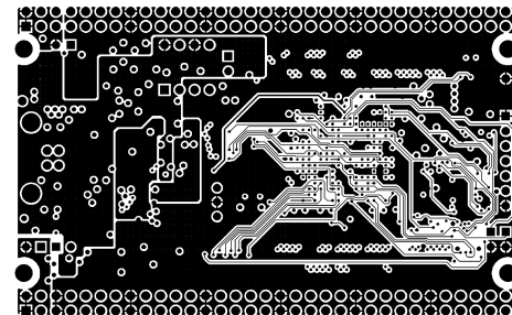
MID LAYER1
