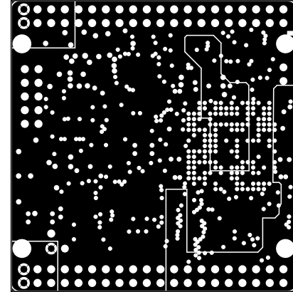
InternalPlane2 (Scale 1:1)
