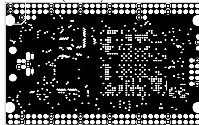
InternalPlane2 (Scale 1:1)
