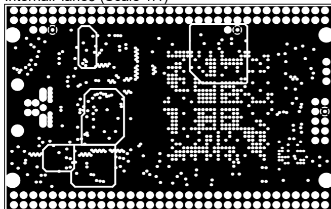
InternalPlane3 (Scale 1:1)
